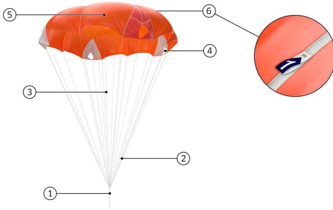
Obr. 1 Přehledový nákres: pohled z espodu.
